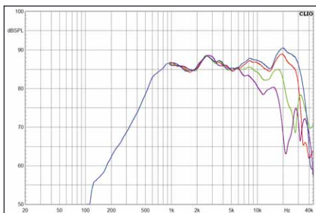
Der Hochtöner ist sehr tief ankoppelbar, ab 2 kHz ist er problemlos im Rennen. Auch er zeigt sich mit einer oberen Grenzfrequenz von 30 kHz sehr breitbandig
