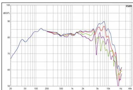
Der Tieftöner läuft bis 4 kHz ohne Störung uns ist damit uneingeschränkt zweiwegetauglich. Mit 84 dB ist er wie viele gute Lautsprecher nicht allzu laut an 1 W, doch das richtet die Endstufe
