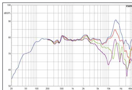
Der Mitteltöner ist ab 150 Hz voll dabei und läuft nach oben aus unserem Messbereich. Erst um 15 kHz macht sich eine ausgeprägte Membranresonanz breit, die mit DSP-Hilfe gefiltert werden muss
