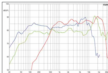
Bereits Tief- und Hochtöner zeigen einen breiten gemeinsamen Frequenzbereich. Der Mitteltöner lässt sich ab 150 Hz mit beliebigen Trennfrequenzen abkoppeln
